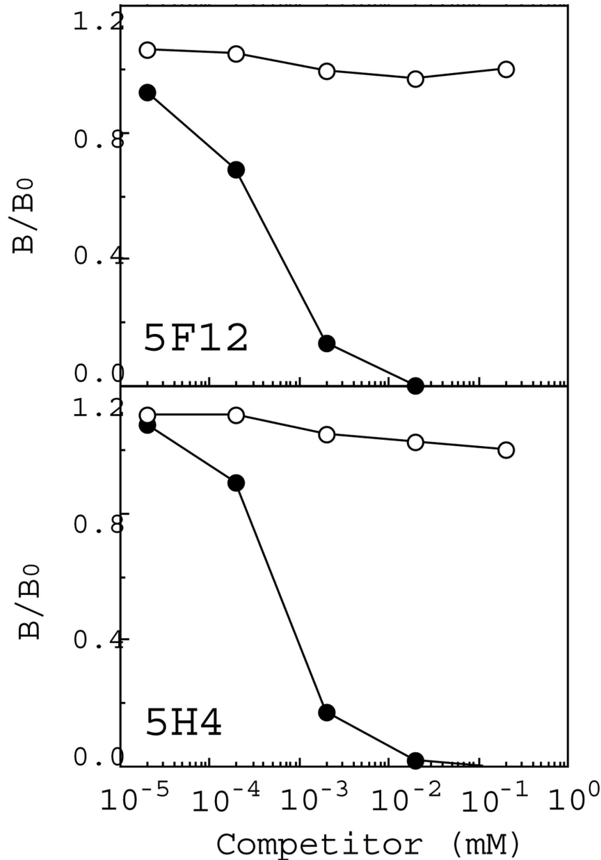
Titration
